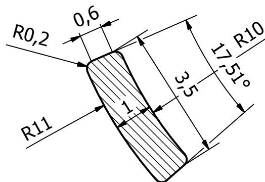
B-B ( 10 : 1 )
