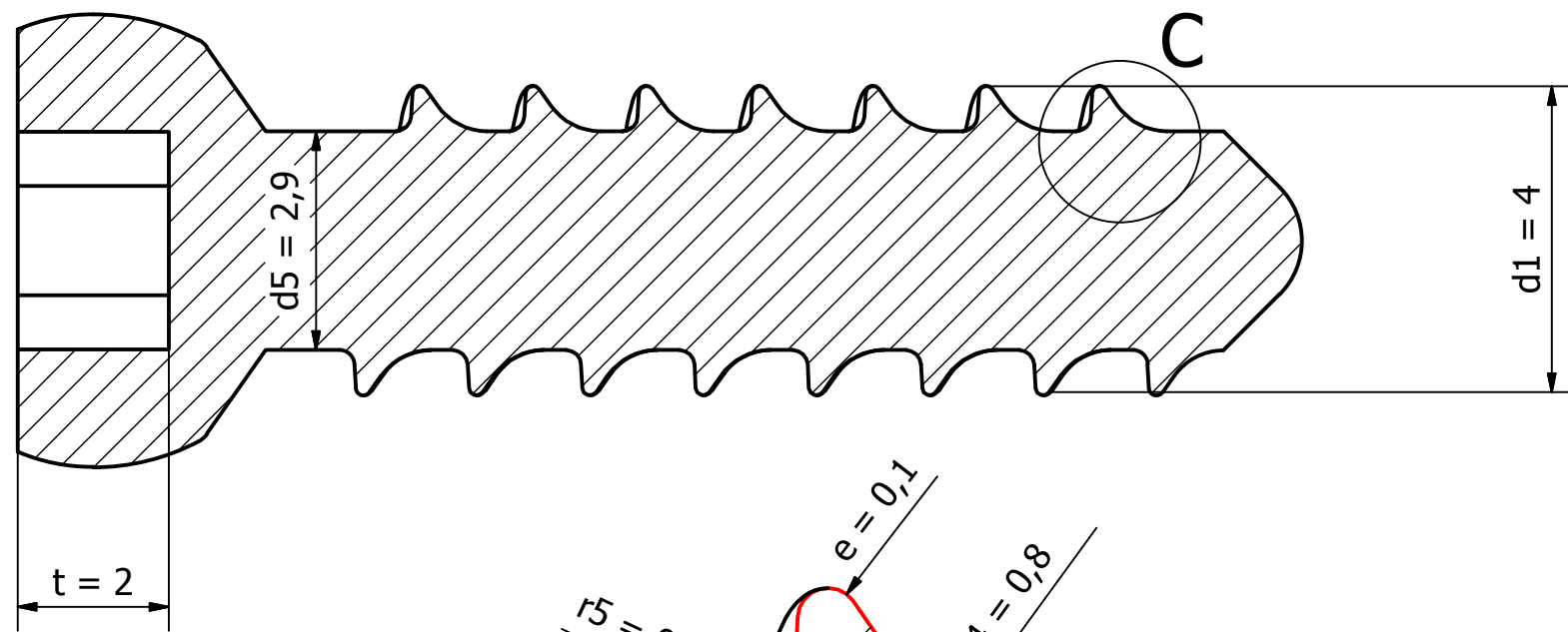
B-B ( 10 : 1 )
